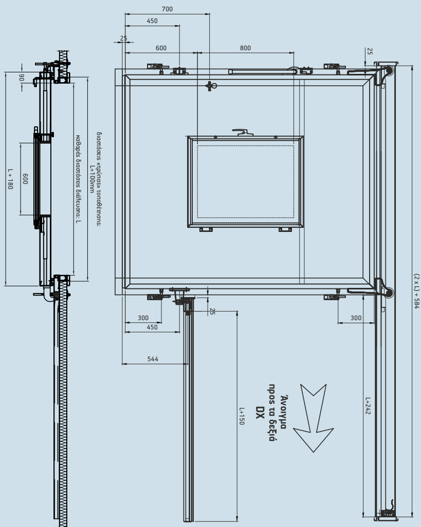
ΚΛΕΙΣΤΡΟ ΜΕ ΚΛΕΙΔΑΡΙΑ ΠΑΡΑΘΥΡΟΥ
