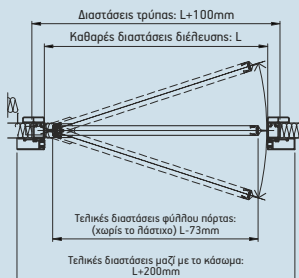
Άνοιγμα προς τα αριστερά SX
