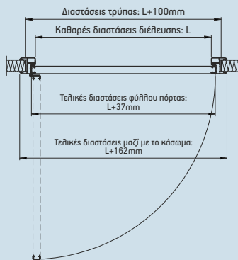
Άνοιγμα προς τα αριστερά SX
