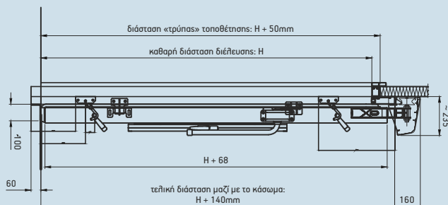
ΕΣΩΤΕΡΙΚΟ ΚΛΕΙΣΤΡΟ ΑΣΦΑΛΕΙΑΣ ΠΑΡΑΘΥΡΟΥ
