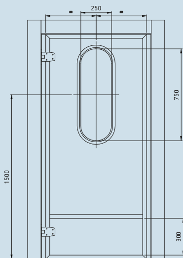
Άνοιγμα προς τα αριστερά SX
