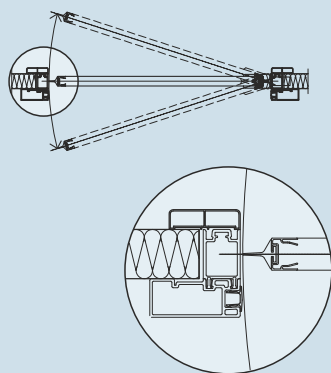
Άνοιγμα προς τα δεξιά DX
